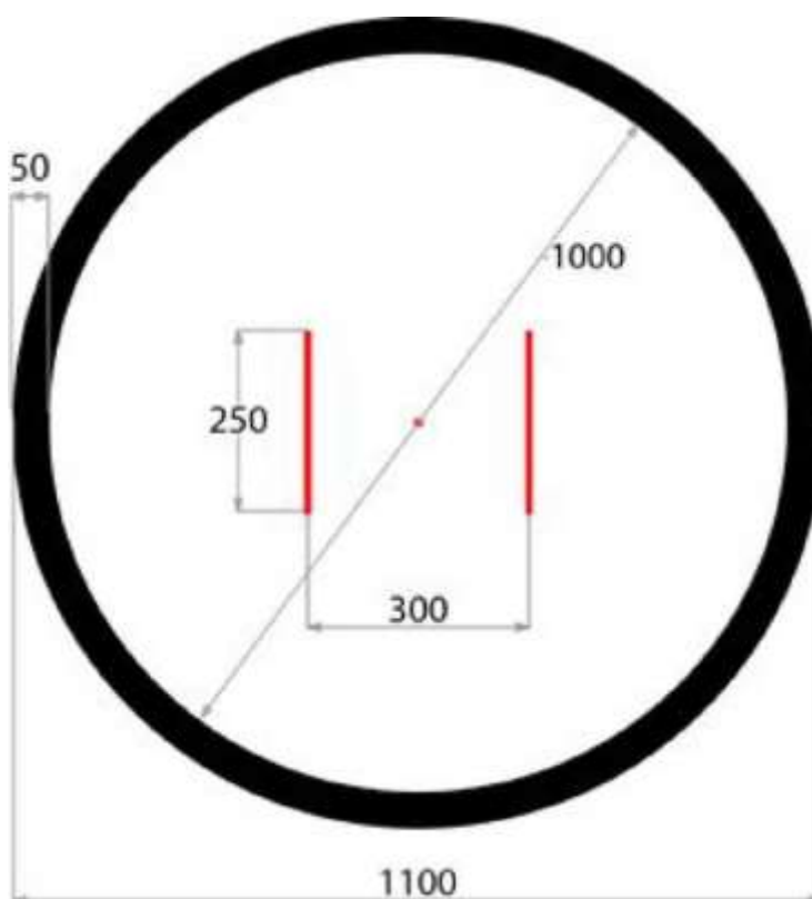
Рис. 2.1. Общий вид поля с размерами
